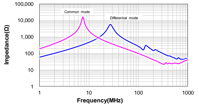
CSUC1514-360M:360M
