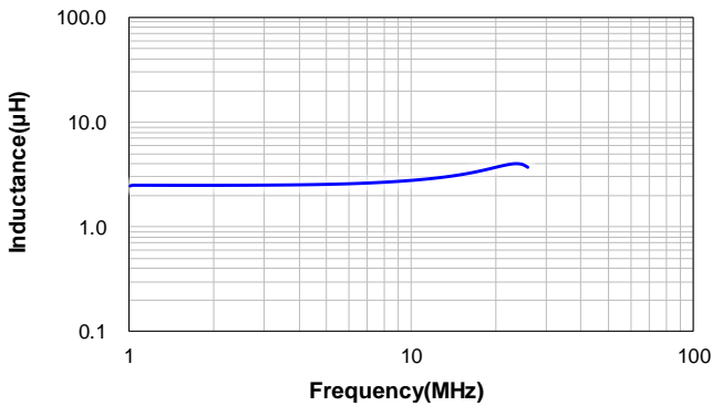
CSUC1514-5R0M:5R0M
