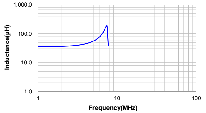
CSUC1514-360M:360M
