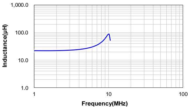
CSUC1514-220M:220M
