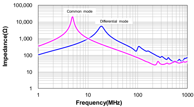
CSUC1514-620M:620M
