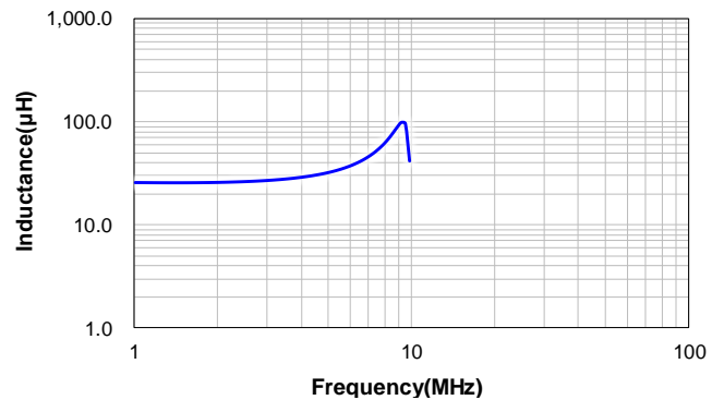
CSUC1514-250M:250M
