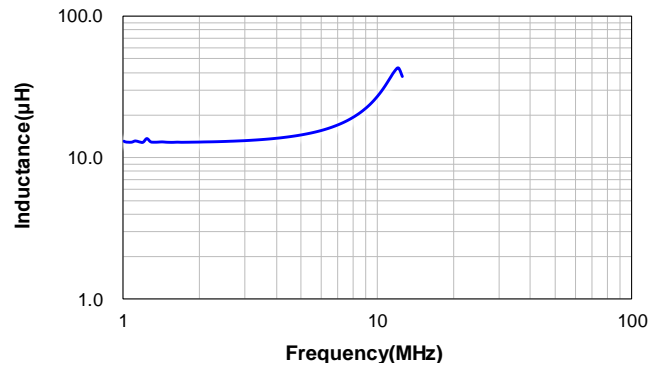
CSUC1514-180M:180M
