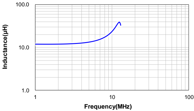
CSUC1514-150M:150M
