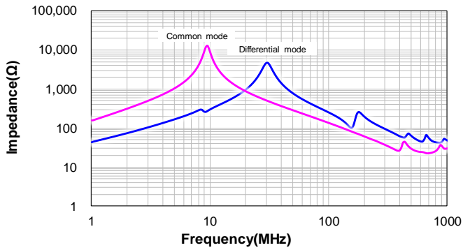
CSUC1514-620M:620M
