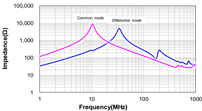
CSUC1514-220M:220M
