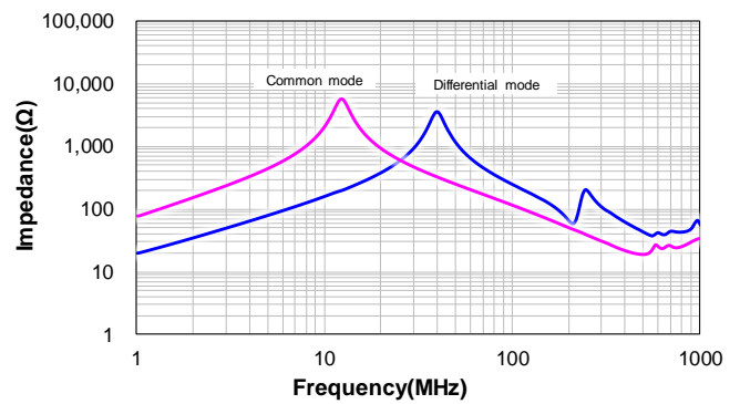
CSUC1514-180M:180M
