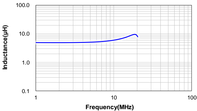
CSUC1514-5R0M:5R0M
