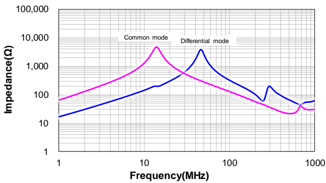
CSUC1514-150M:150M
