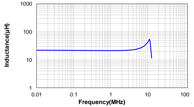
CSBX1812-330M
