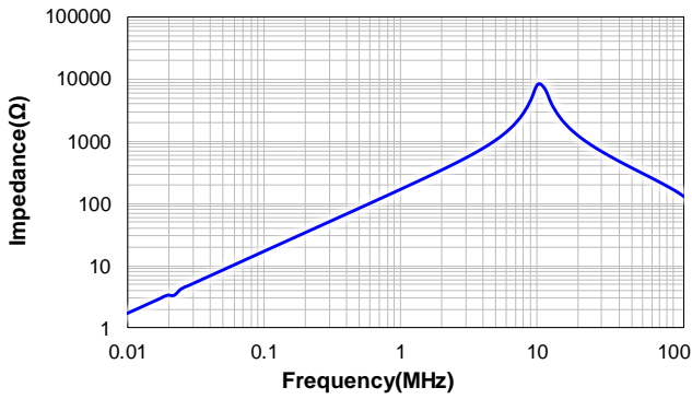
CSBX1812-270M
