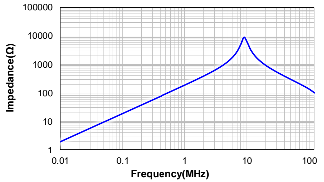
CSBX1812-330M
