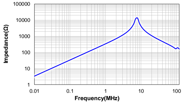
CSBX1812-560M
