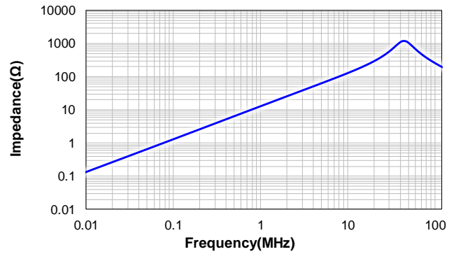
CSBX1812-4R3M
