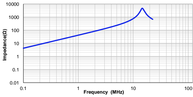
VSEG1060-6R8M
