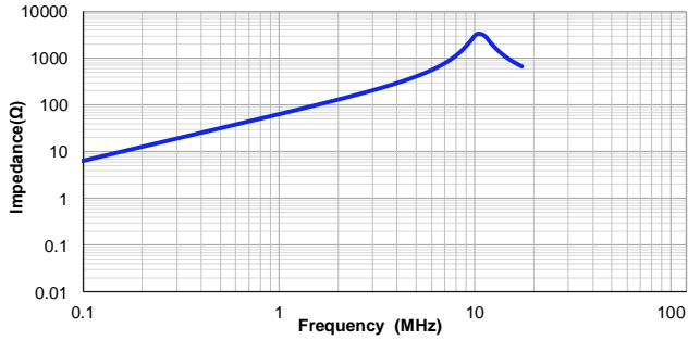
VSEG1060-100M
