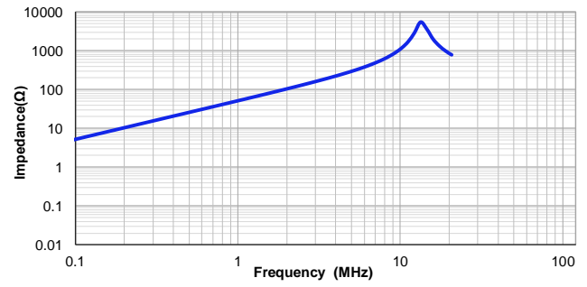
VSEG1060-8R2M
