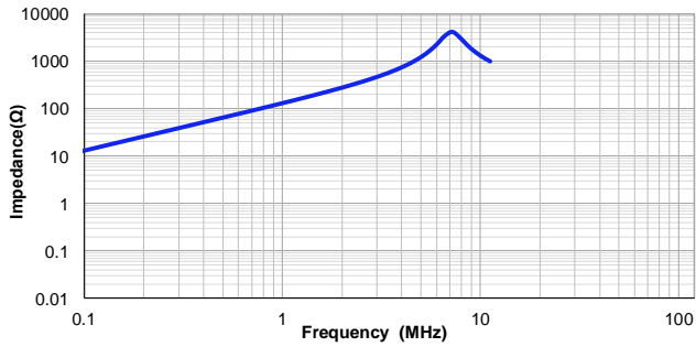
VSEG1010-220M
