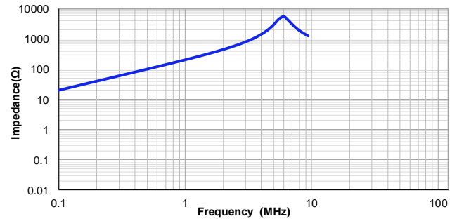
VSEG1010-330M
