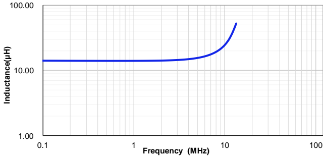
VSEG0550H-150M
