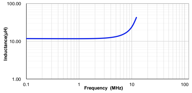
VSEG0550H-120M
