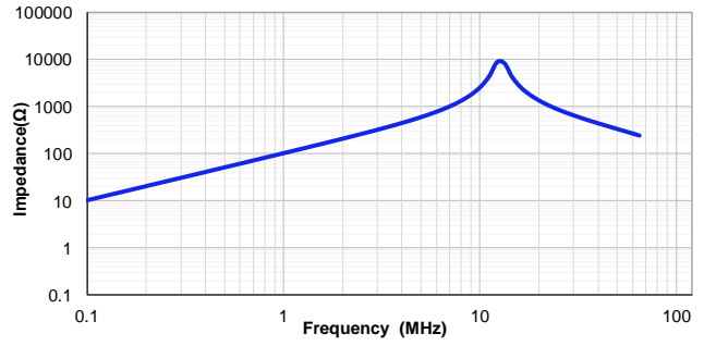
VSEG0550H-180M
