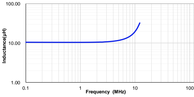
VSEG0550H-100M
