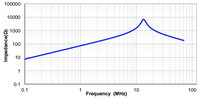
VSEG0550H-120M
