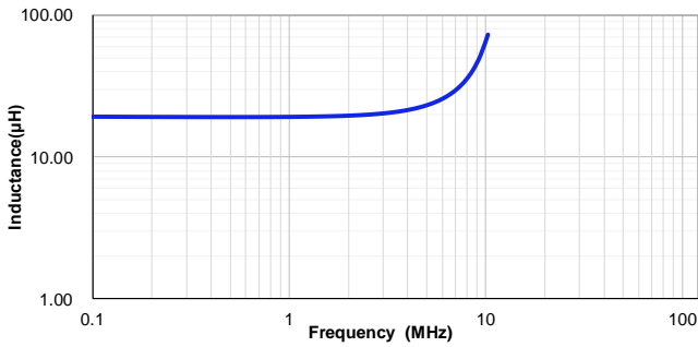
VSEG0550H-220M
