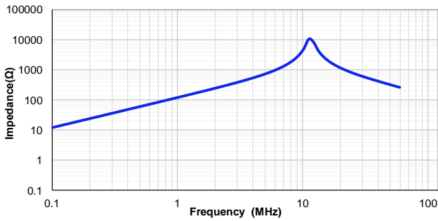
VSEG0550H-220M
