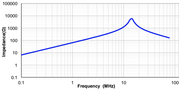
VSEG0550H-100M
