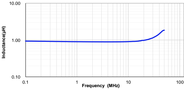
VSEB0770-R80M
