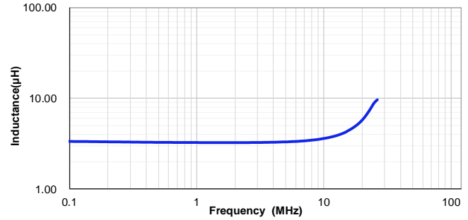
VSEB0770-3R3M
