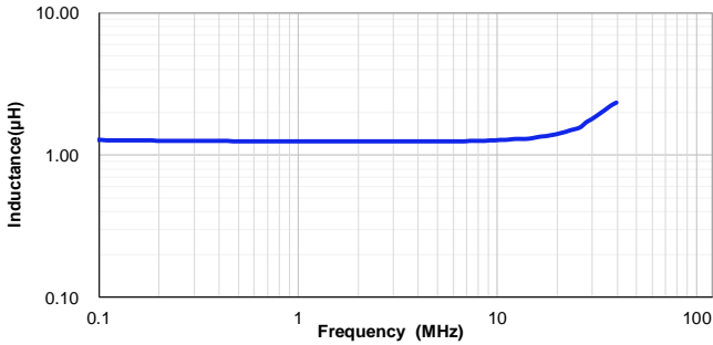
VSEB0770-1R2M
