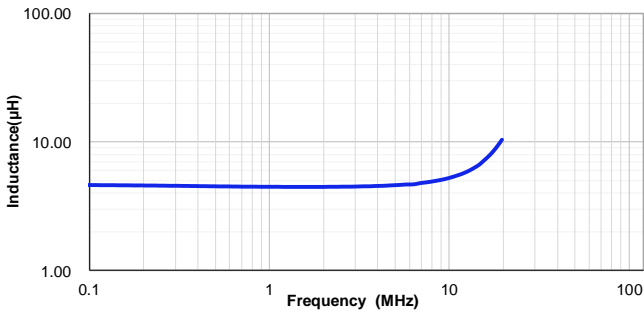
VSEB0770-4R7M
