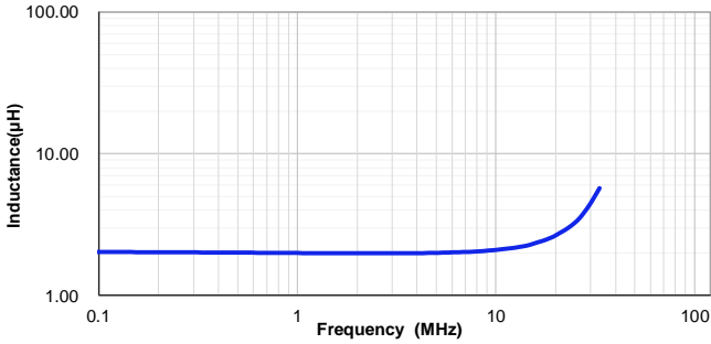
VSEB0770-2R2M
