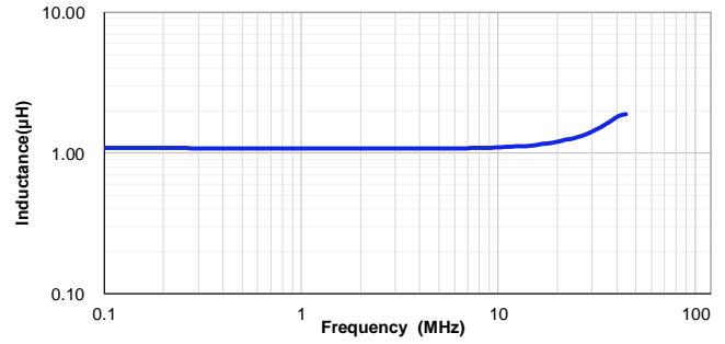
VSEB0770-1R0M
