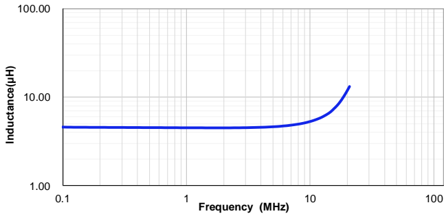
VSEB0730-4R7M
