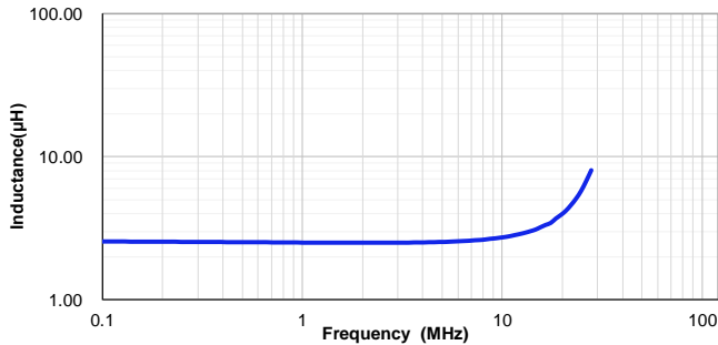
VSEB0730-2R7M
