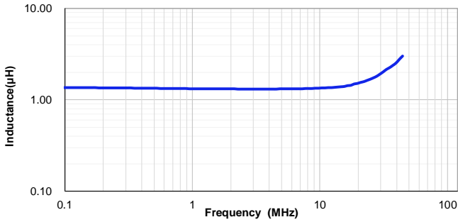
VSEB0730-1R5M
