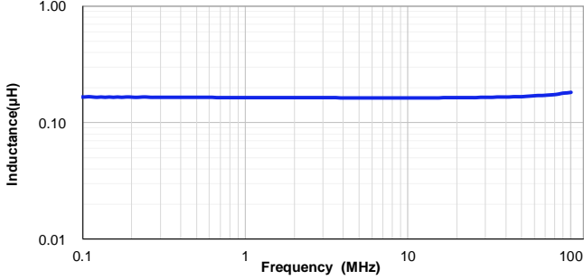
VSEB0730-R16M
