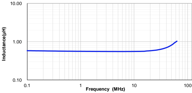
VSEB0730-R60M
