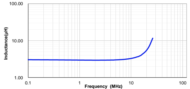
VSEB0730-3R3M
