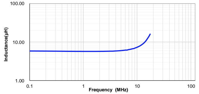
VSEB0730-5R6M
