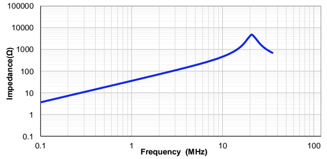
VSEB0730-5R6M
