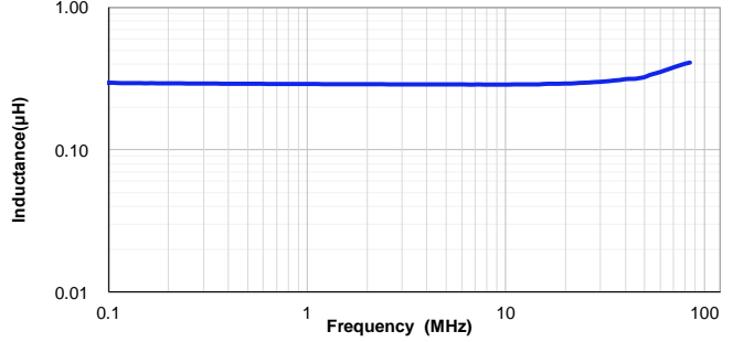
VSEB0730-R30M
