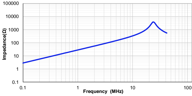
VSEB0730-4R7M
