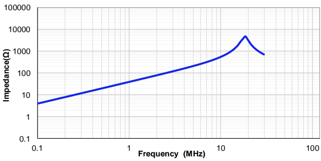
VSEB0730-6R8M
