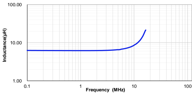
VSEB0730-6R8M
