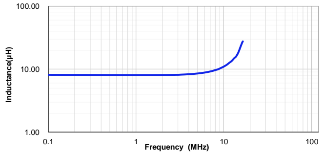
VSEB0660-8R2M
