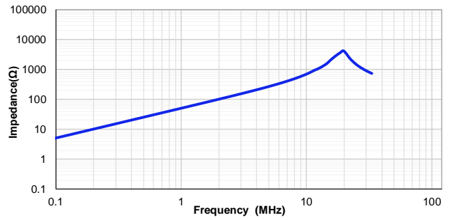
VSEB0660-8R2M
