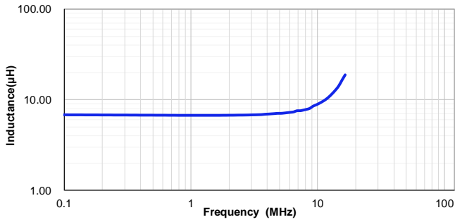
VSEB0660-6R8M
