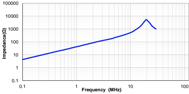
VSEB0660-6R8M
