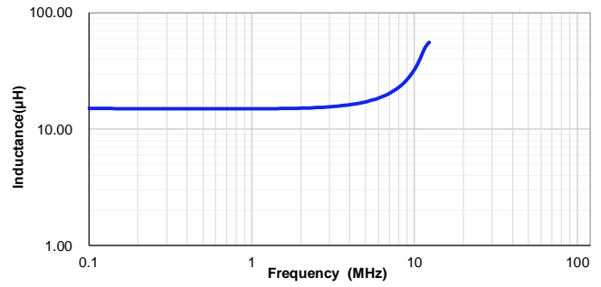
VSEB0660-150M
