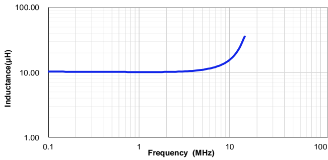
VSEB0660-100M
