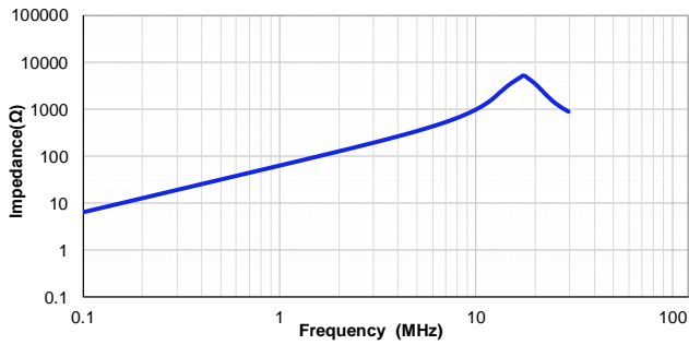
VSEB0660-100M
