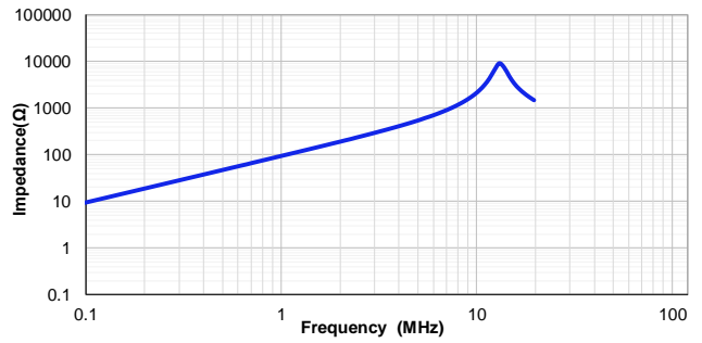
VSEB0660-150M
