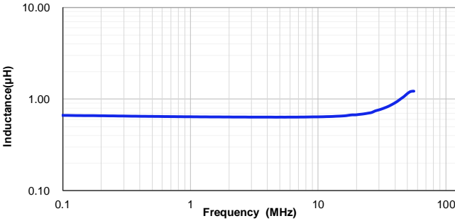
VSEB0630-R68M
