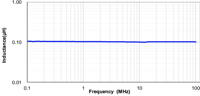
VSEB0630-R18M
