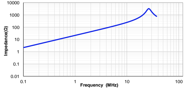
VSEB0630-3R3M
