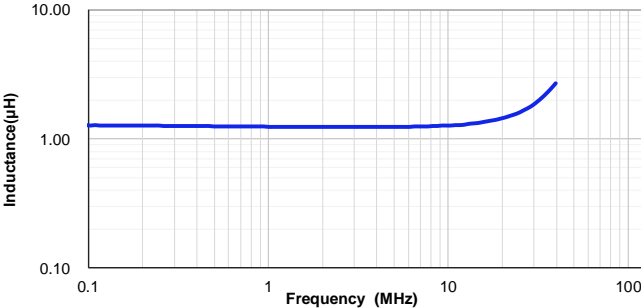
VSEB0630-1R2M
