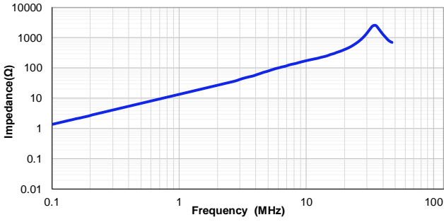
VSEB0630-2R2M
