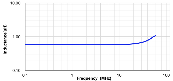
VSEB0630-R56M
