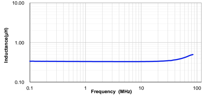
VSEB0630-R33M
