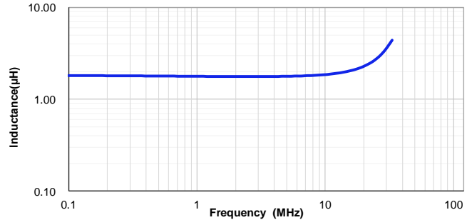
VSEB0630-1R8M
