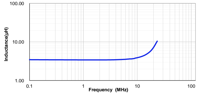
VSEB0630-3R3M
