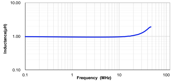
VSEB0630-1R0M
