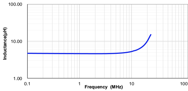
VSEB0630-4R7M
