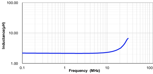
VSEB0630-2R2M
