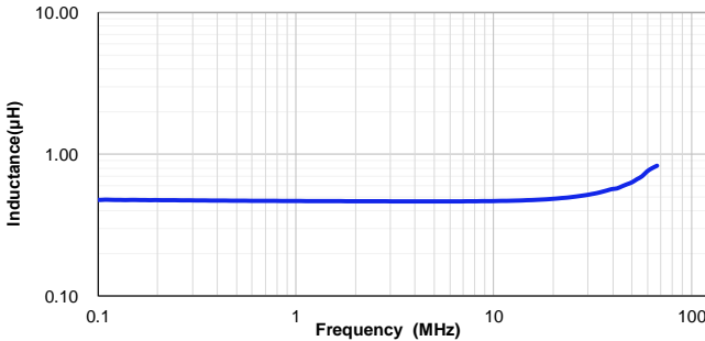
VSEB0630-R47M
