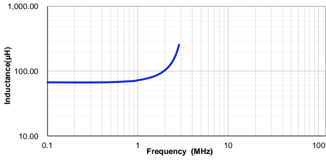
VSAB1365-680M
