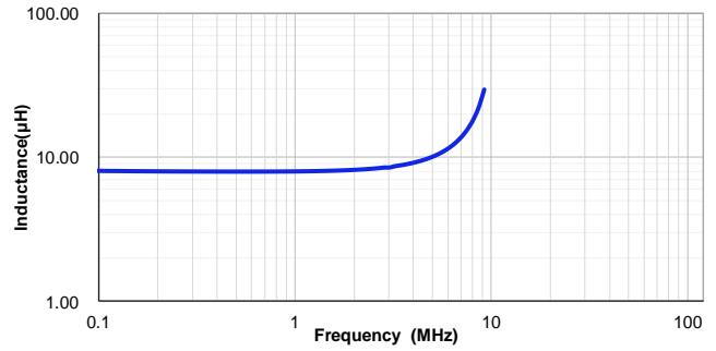
VSAB1365-8R2M
