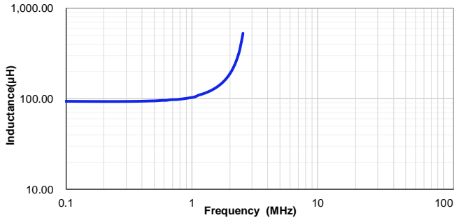
VSAB1365-101M
