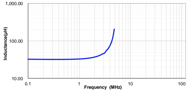
VSAB1365-330M
