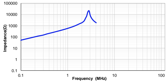
VSAB1365-820M
