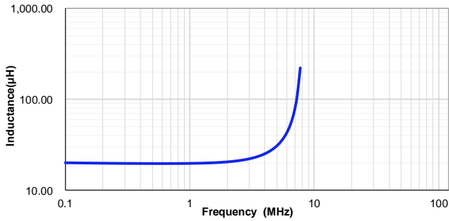
VSAB1365-220M
