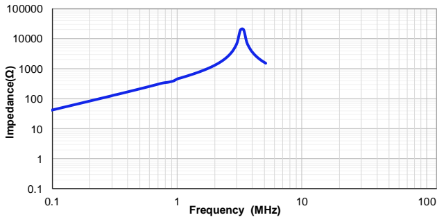
VSAB1365-680M
