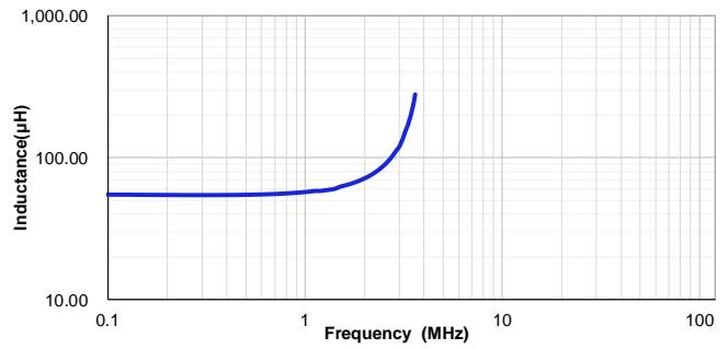
VSAB1365-560M
