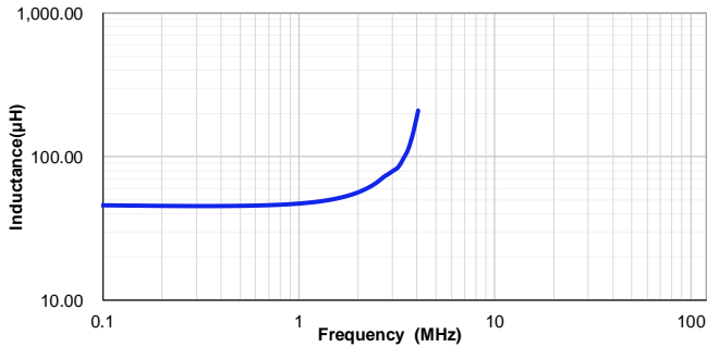
VSAB1365-470M
