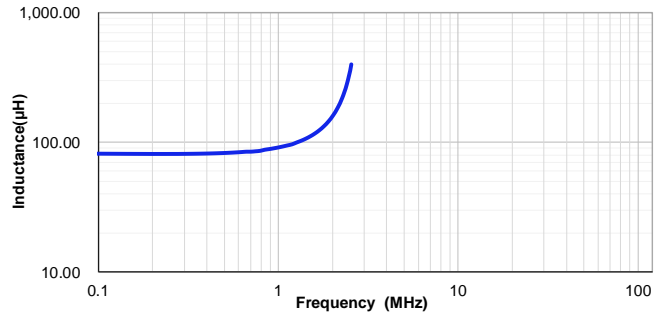
VSAB1365-820M
