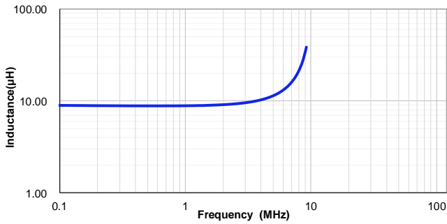
VSAB1365-100M
