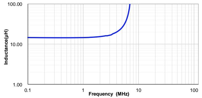
VSAB1365-150M
