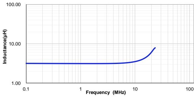
CSEG0520H-3R3M
