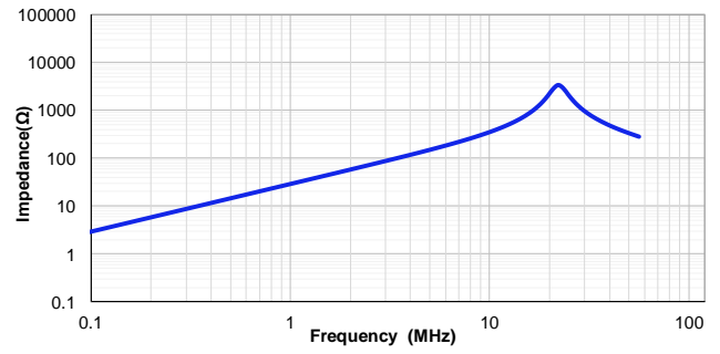
CSEG0520H-4R7M
