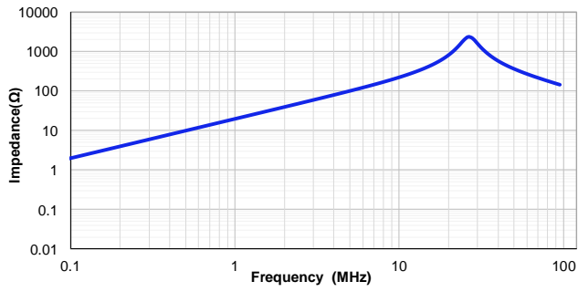
CSEG0520H-3R3M
