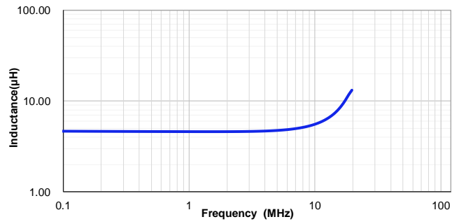
CSEG0520H-4R7M
